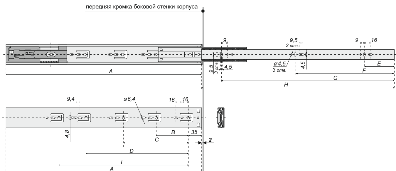
СХЕМА ПРИСАДКИ НАПРАВЛЯЮЩИХ
